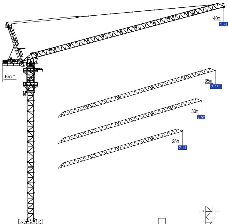
固定式 Stationary
